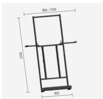
Platten-Pritsche
